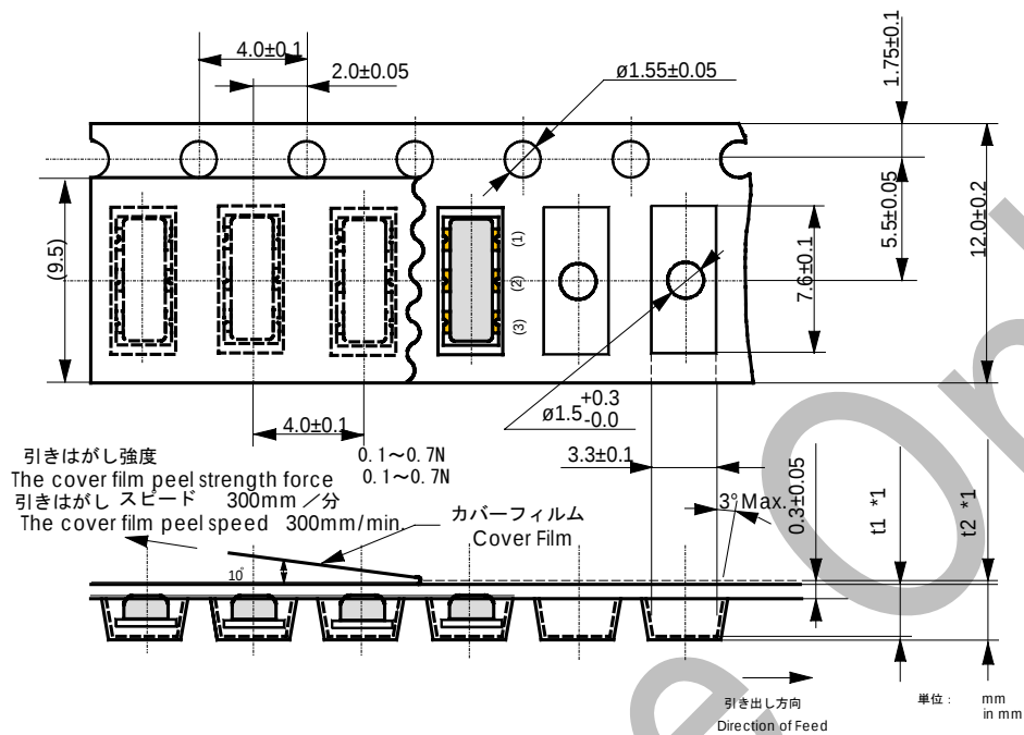
第3図 プラスチックテープの外形寸法図 Figure 3. Dimensions of Plastic Tape (CSTCC2M00G53-R0)
