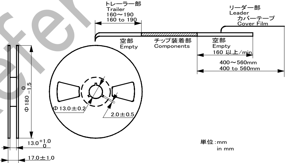
第4図 プラスチックリールの外形寸法図 Figure 4. Dimensions of Plastic Reel (CSTCC2M00G53-R0)
