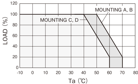
HWS50
