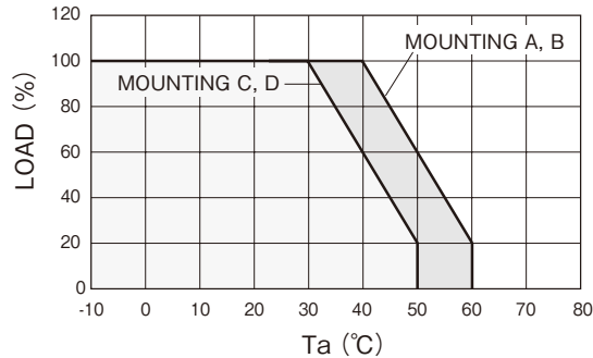
HWS50/A
