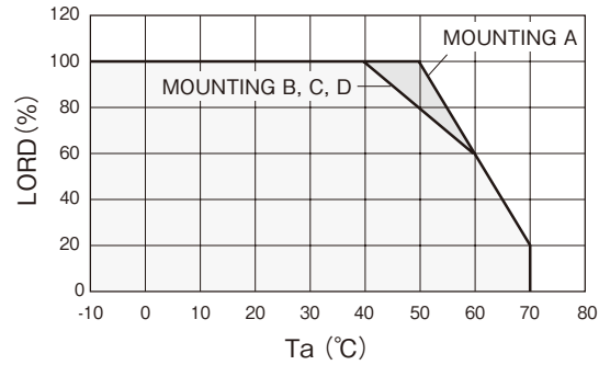
HWS100
