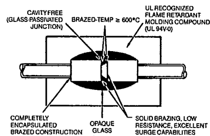
FIG. 6 — SUPERECTIFIER
